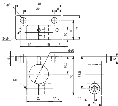
Bracket • φ20
